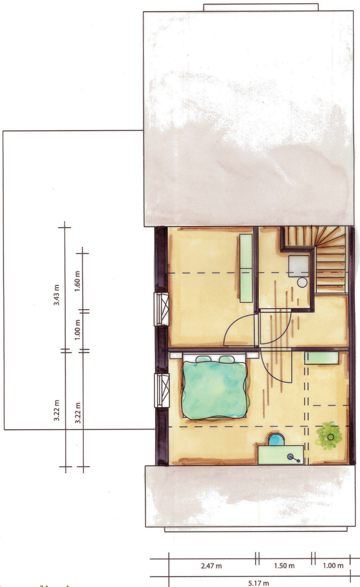
1e verdieping
